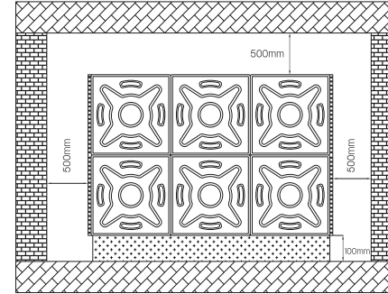
Karşıdan Görünüm
