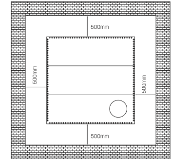
Üstten Görünüm
